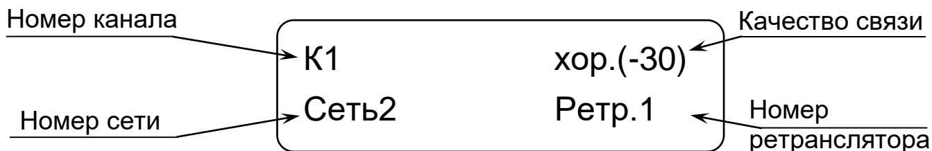
Рисунок 12 – Окно индикации состояния радиосети
