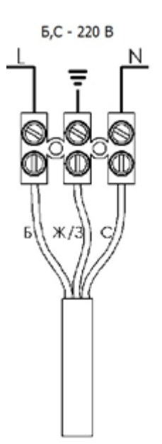
Рис. 2. Схема подключения LCL40PP/40S1
