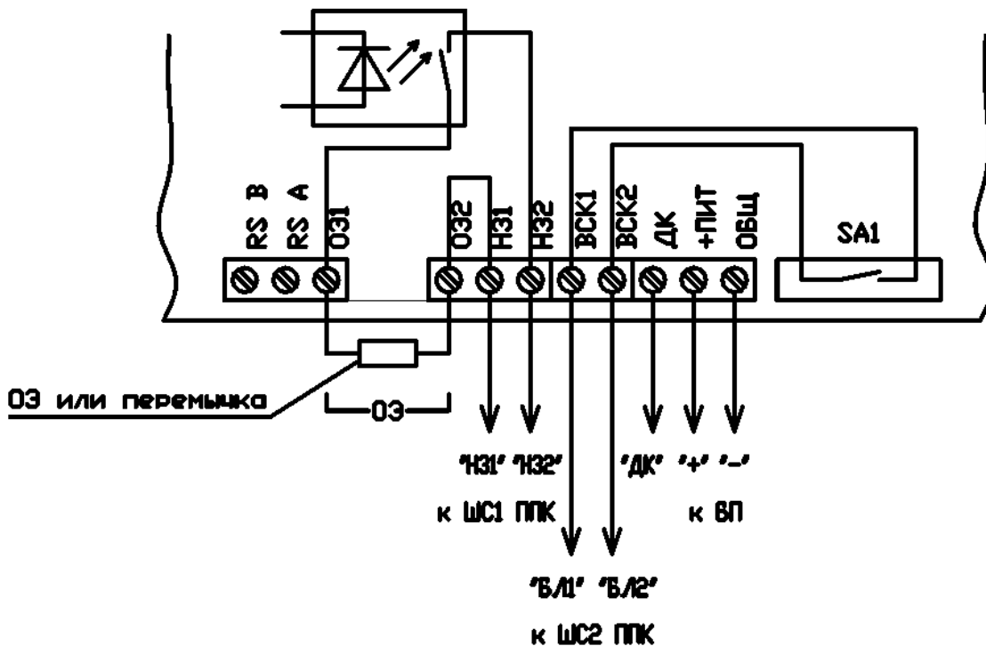
Рисунок В.1 – Подключение к двум шлейфам сигнализации
