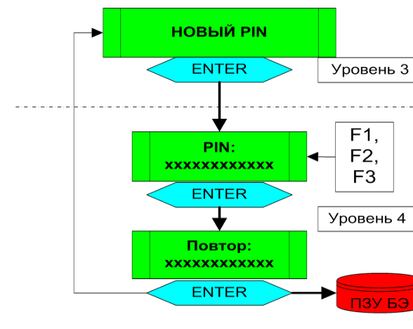
Рис. 3.4. Структурная схема раздела «НОВЫЙ PIN» системного меню ПУ
