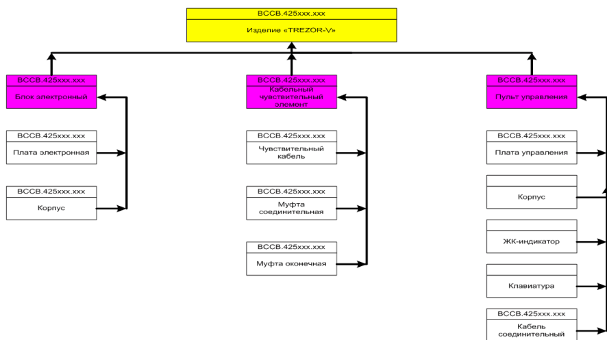
Рис. 2.1. Схема деления изделия «TREZOR-V» на составные части
