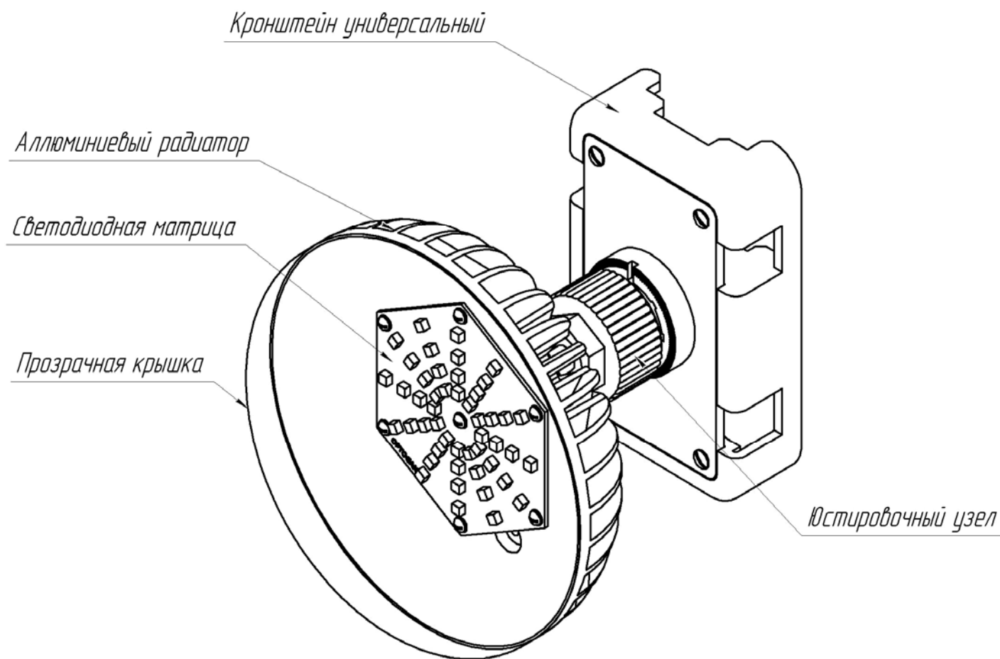
Рисунок 1.1 – Фонарь. Внешний вид
